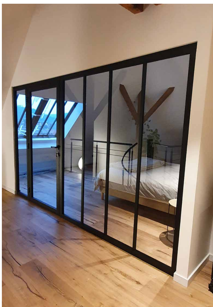
Cloison sur mesure type Atelier avec porte battante Vitrage phonique / acoustique
